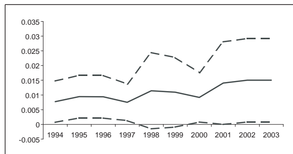
Output Gap Coefficient \pm 2 SE
